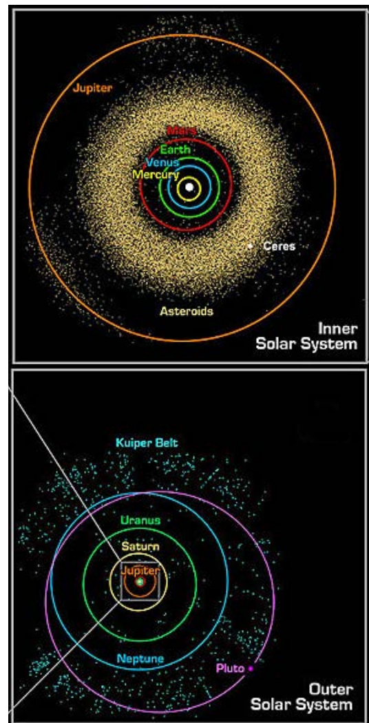
Položaj glavnog asteroidnog pojasa i Ceres u Sunčevom sustavu
