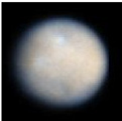
Ceres kako ju je snimio teleskop Hubble...
