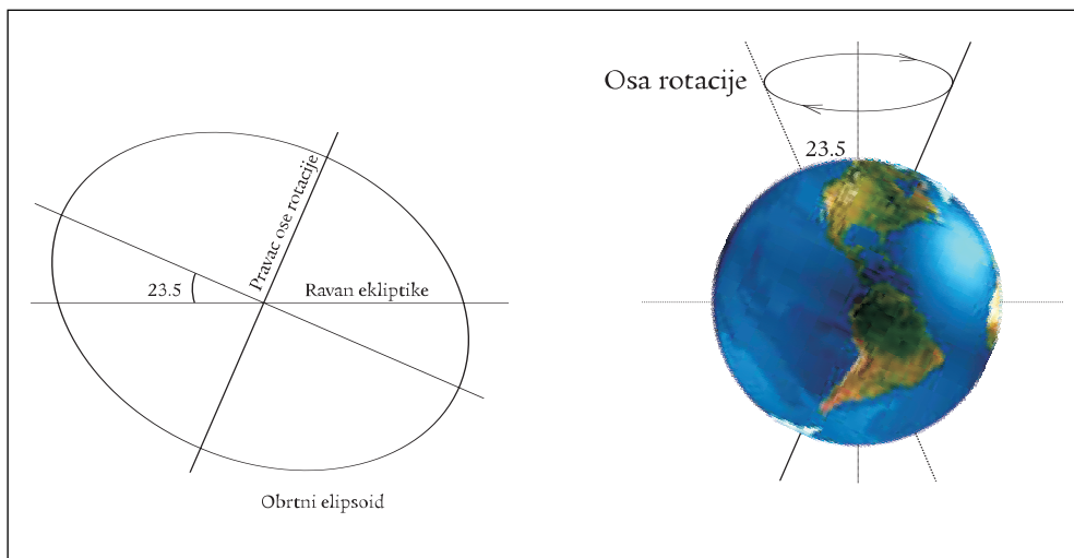
Slika#4 – Precesija
